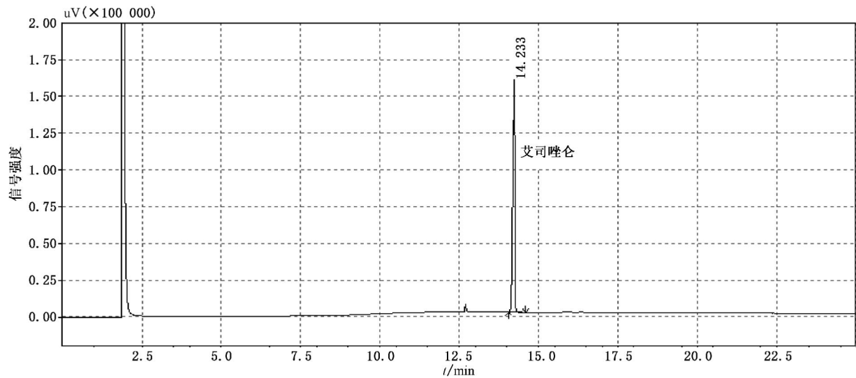
图 B.1 艾司唑仑气相色谱图
