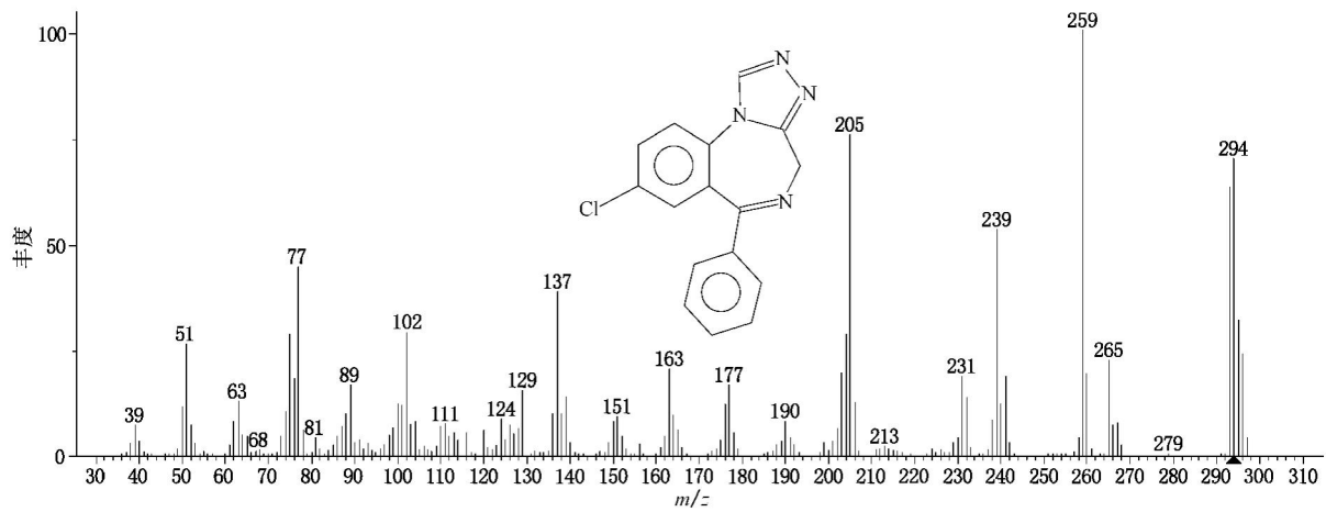
图 B.2 艾司唑仑质谱图
