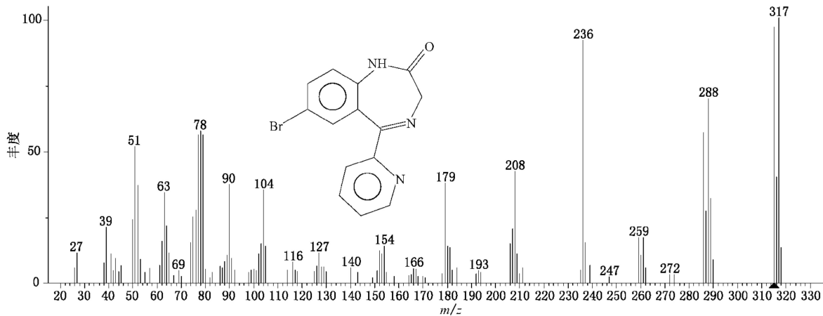
图 B.2 溴西洋质谱图
