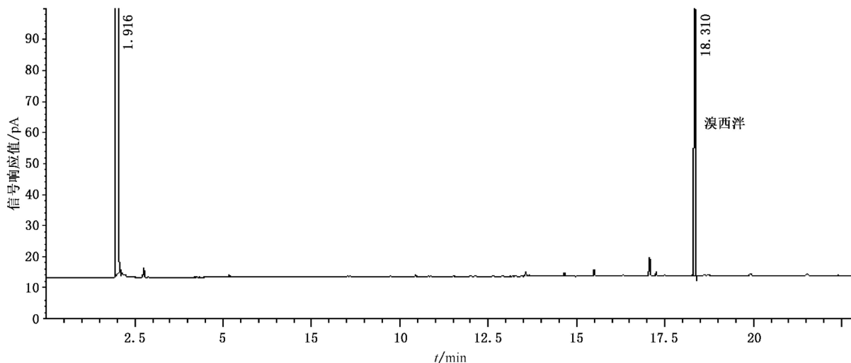
图 B.1 溴西洋气相色谱图
